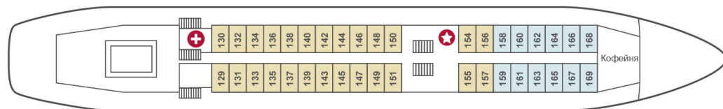
Главная палуба
